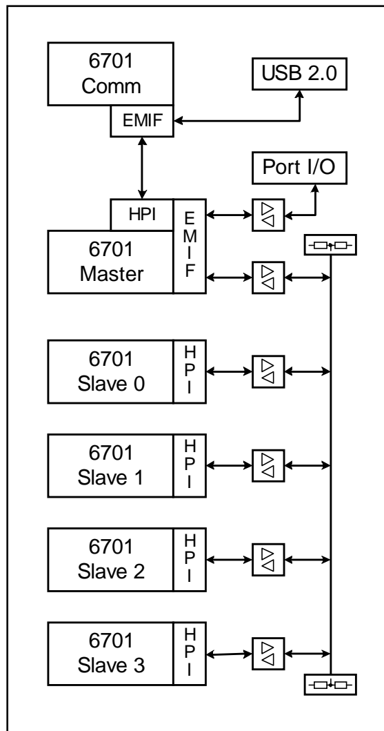
Abb. 1: Grundstruktur
