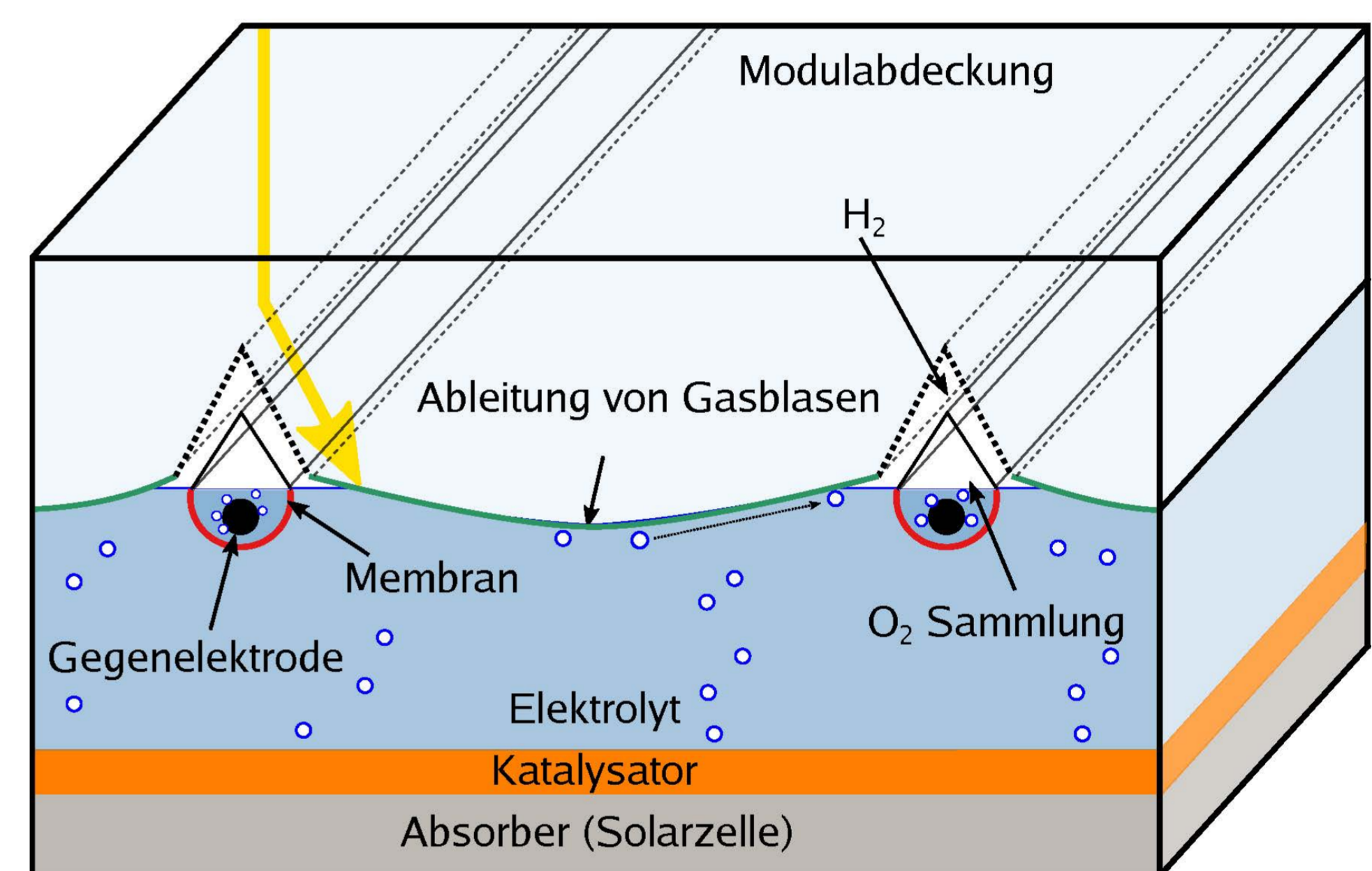
Bild 2: Prinzip der photoelektrochemischen Zelle
