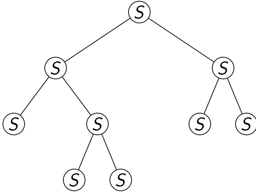
ein S -Ableitungsbaum
