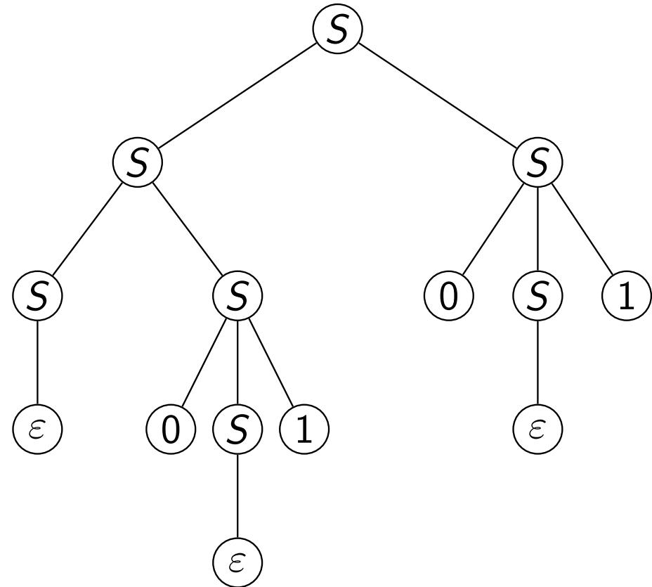
ein vollständiger S -Ableitungsbaum
