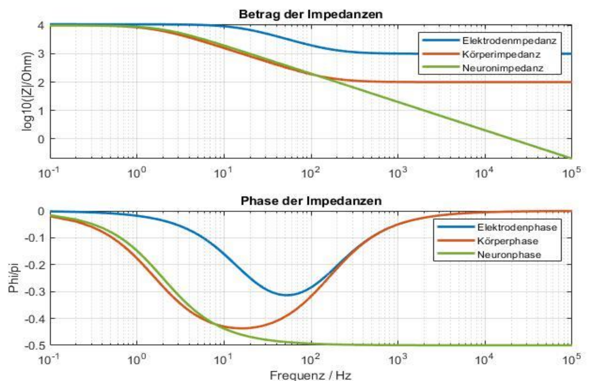
Abb. 2: Bode-Diagramm der wichtigsten Impedanzen von Elektroden und Körper
