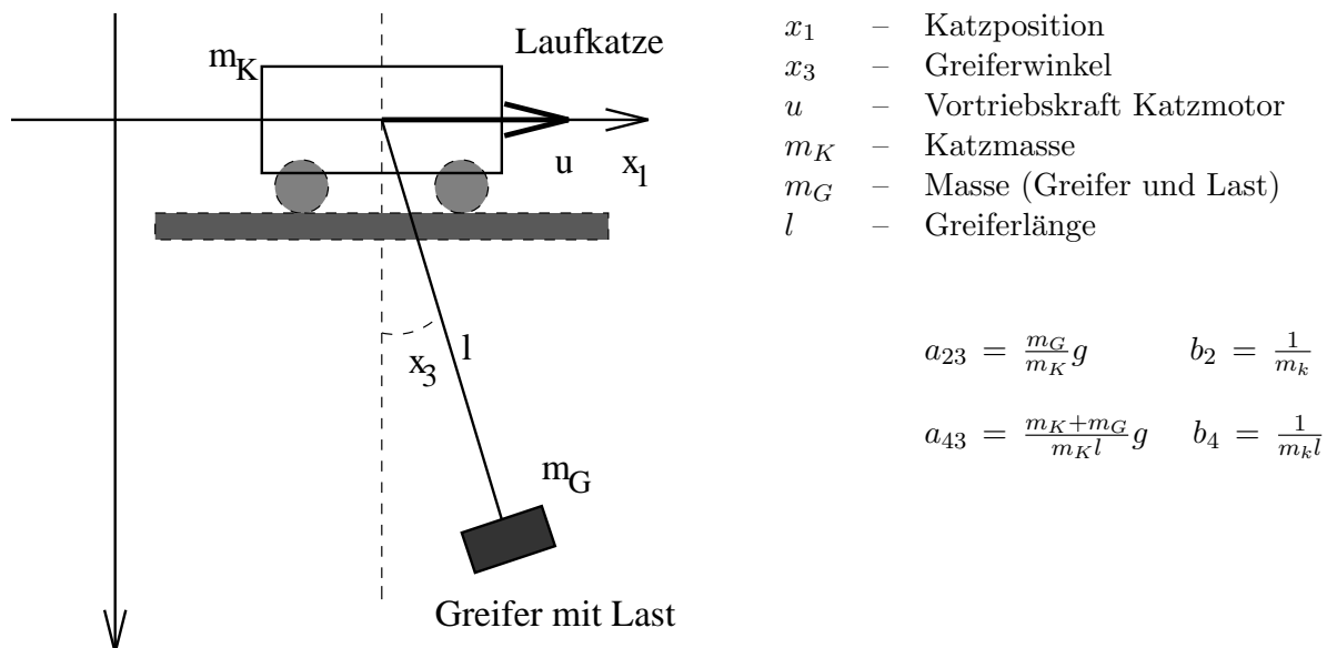
Abbildung 1: Verladebrücke
