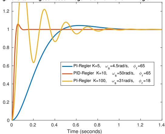
Sprungantworten im geschlossenen Regelkreis mit PI- und PID-Regler
