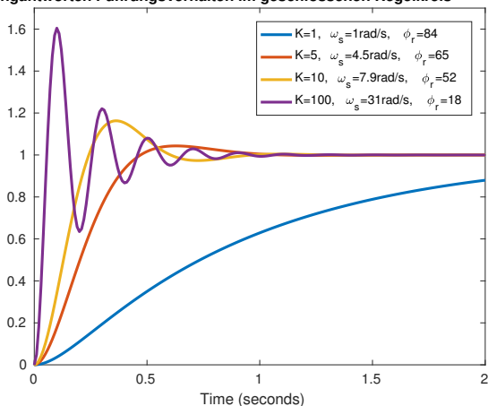
Sprungantworten Führungsverhalten im geschlossenen Regelkreis
