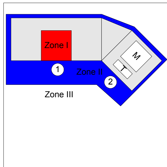
Bild 1: Versuchsraum nach DIN 5053-7
