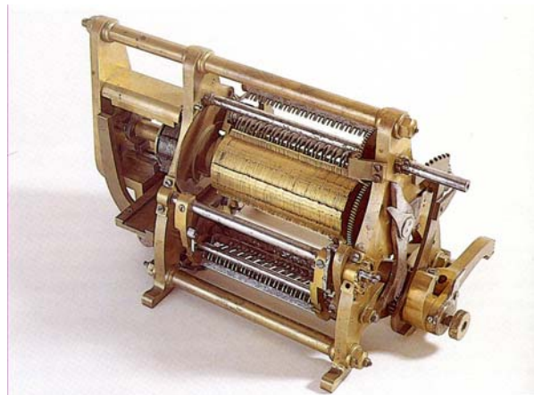
Abb.3: Die Differenzenmaschine von Wiberg
