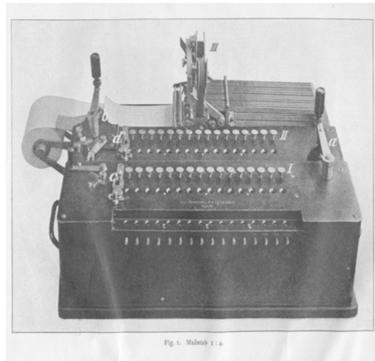
Abb. 4: Die Differenzenmaschine von Hamann
