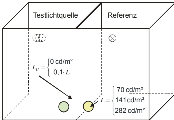
Abbildung 9: Schematische Darstellung des Versuchsaufbaus links und Überblick über die Versuchsparameter rechts [3]
